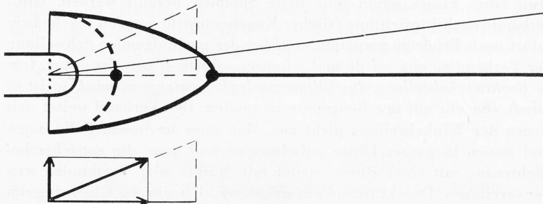
Abb. 1. Gestrichelte Linie: Kurzer Bügel, kurzer Zug. Eine Verschiebung des Patienten nach der Seite hat eine grosse Richtungsänderung des Zuges (siehe Winkel!), eine starke Verschiebungsgefahr des Drahtes und eine (nicht gezeichnete!) Drehung des Bruchstückes zur Folge. — Ausgezogene Linie: Langer Bügel, langer Zug; meidet bei gleicher Verschiebung alle drei Gefahren fast vollständig. — Unten: Kräfteparallelogramm bei schlechtem, kurzem Zug: Ein Teil des Zuges missbraucht sich zum Verschieben des Drahtes.
