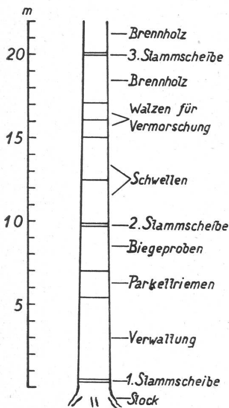
Abbildung 12. Schema der Aufarbeitung der sogen. A-Stämme.
