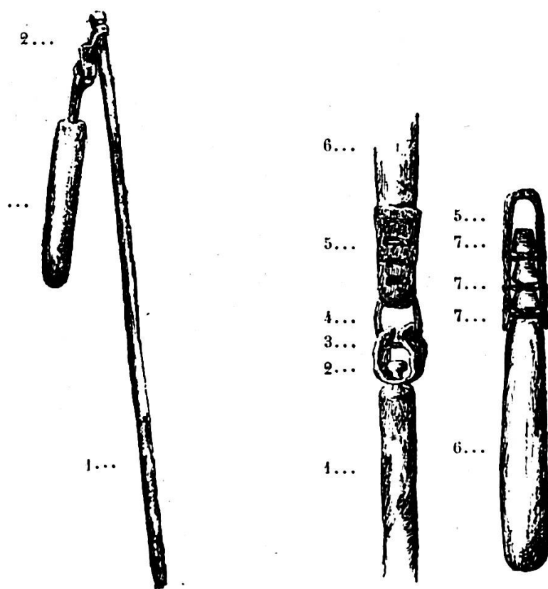
FIG. 2. Fléau valaisan (Evolène): 1. māxso . — 2. kōrāyē . — 3. vērzé . FIG. 3. Fléau genevois (Bernex): 1. lyuāzama . — 2. nyuè . — 3. tōrnè . — 4. antralā (Dardagny). — 5. ḡapa . — 6. varḡā . — 7. ākōḡ .
