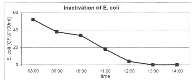
Abbildung: Abbau von E. coli mit zunehmender Expositionszeit der 1,5-Liter-PET-Flasche
