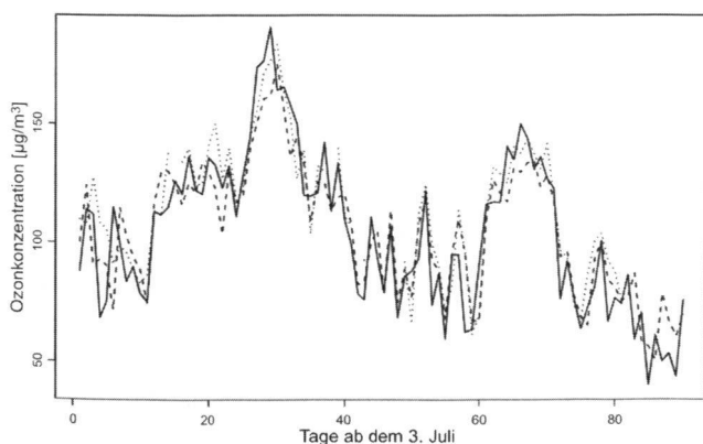
Abbildung 1: Vergleich zwischen der Ozonprognose basierend auf gemessenen resp. prognostizierten Werten der meteorologischen Parameter mit den in Etzelkofen gemessenen Ozonwerten des Sommers 2004. Die ausgezogene Linie stellt die gemessenen Ozonwerte dar, die unterbrochene Linie die auf Messdaten der Meteoroparameter beruhende Prognose der Ozonwerte und die gepunktete Linie die auf prognostizierten Meteoroparametern beruhende Prognose der Ozonwerte.
