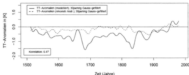
Abbildung: Europäische Jahresmitteltemperaturanomalien von 1500 bis 1990 (Referenzperiode: 1901-1990). Die gestrichelte Kurve stellt die rekonstruierten bzw. instrumentellen Temperaturanomalien dar und die durchgezogene Kurve die modellierten. Beide Kurven wurden mit einem 30-jährigen Gauss-Filter geglättet. Die Korrelation zwischen beiden Kurven beträgt 0.47.
