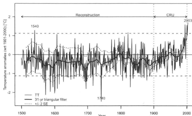
Abbildung 1: Jährliche Temperaturanomalien für die Alpen (TT; Referenzperiode 1901-2000) der Jahre 1500-2003. Die dicke Kurve ist ein 31-Jahresfilter um die niederfrequente Variabilität zu unterstreichen. Die gestrichelten horizontalen Linien sind die \pm 2 Standardabweichungen des zwanzigsten Jahrhunderts. Die fein gestrichelten Linien kennzeichnen die Unsicherheiten der Rekonstruktion ( \pm 2 Standardfehler). Die absoluten Extremjahre sind ausgeschrieben.
