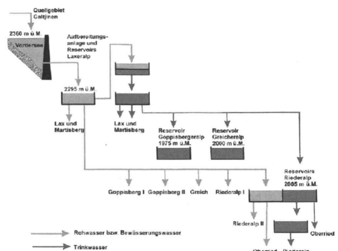
Fig. 2: Schema der Wasserversorgung im Aletschgebiet
