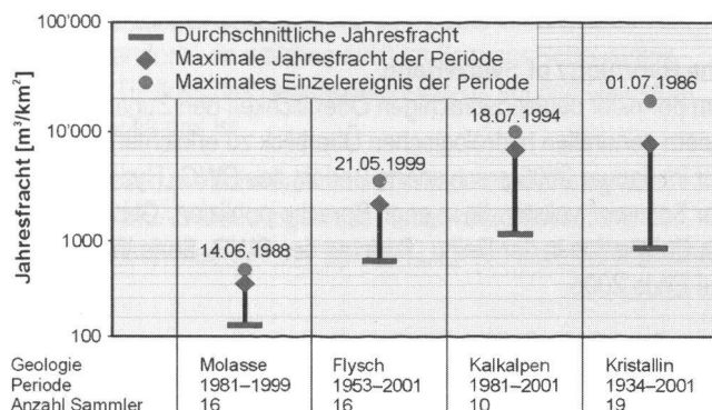
Figur: Feststofffrachten ausgewählter Geschiebesammler, unterteilt nach Geologie.
