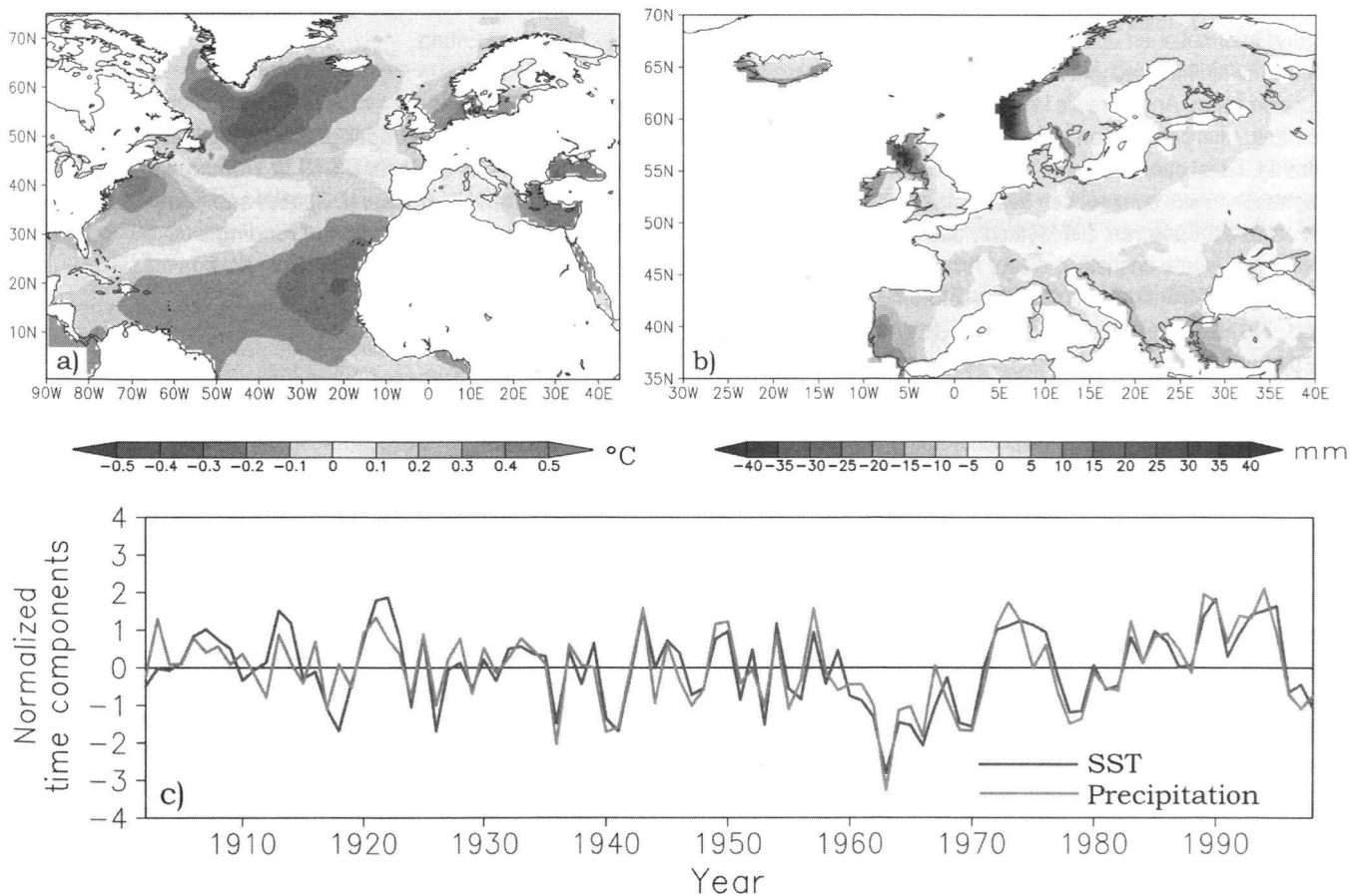
Abbildung 1: CCA 1 für DJFM 1902–1998. a) SST, b) Niederschlag über Europa und c) normierte Zeit-komponenten der SSTs (schwarz) und des Niederschlags (grau). Die Korrelation zwischen den zwei Zeitreihen beträgt 0.87. Die erste CCA Variate erklärt 16% der Niederschlagsvariabilität und 13% der SST Variabilität.
