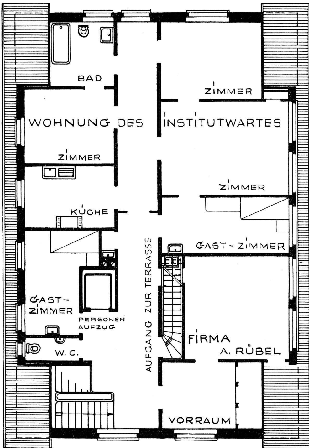
DACHSTOCK
