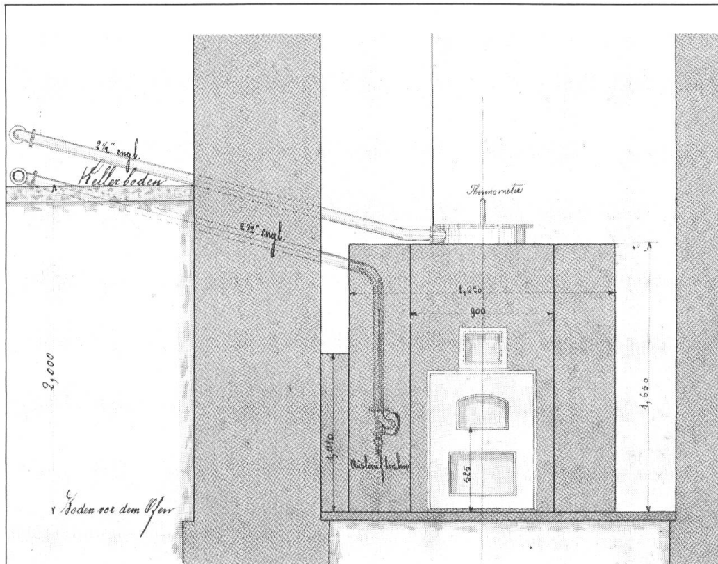
Sulzer-Zentralheizofen für Käsekeller 1880
