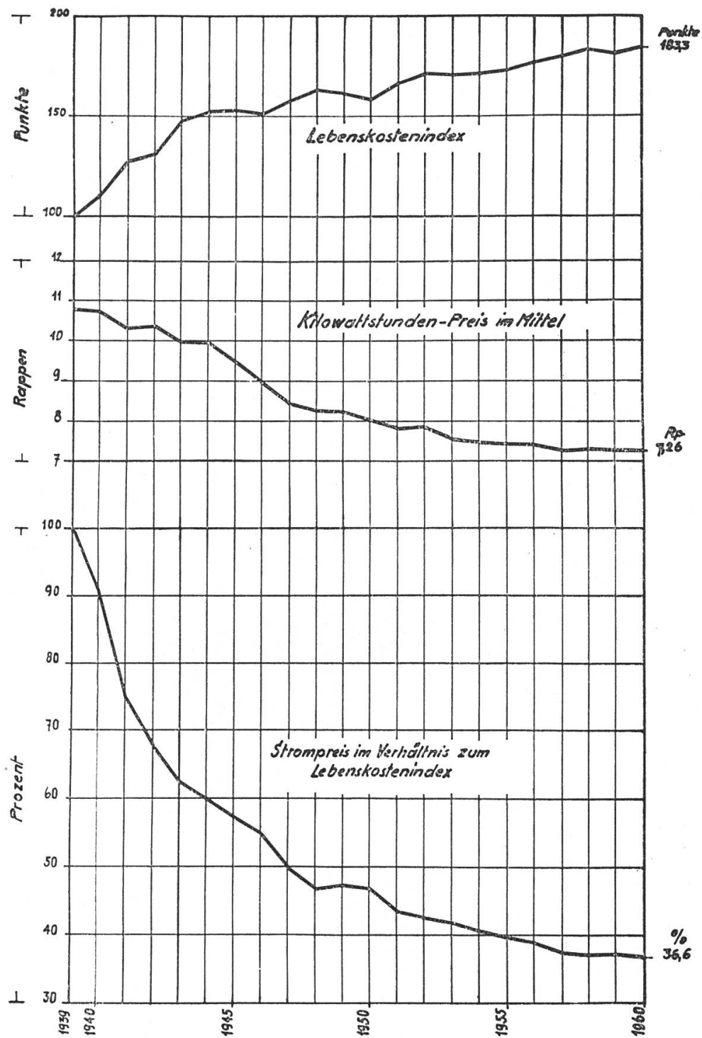
Elektrizitätswerk Burgdorf: Entwicklung des durchschnittlichen Strompreises verglichen mit dem Lebenskostenindex.
