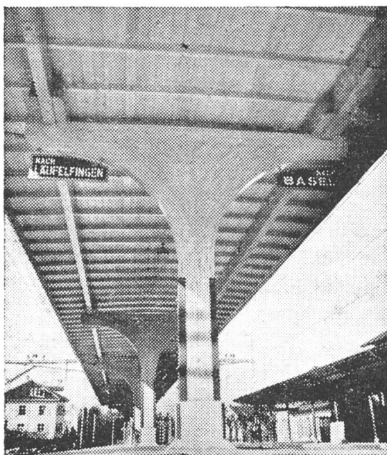
Perrondach S.B.B. Bahnhof Liestal Hetzerkonstruktion ausgeführt durch Gribi & Co. AG.
