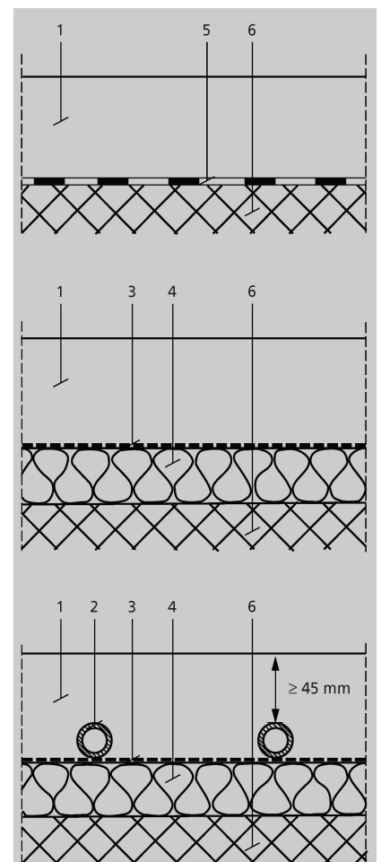
Fig. 1 Structures typiques de chapes flottantes (selon [4]).
