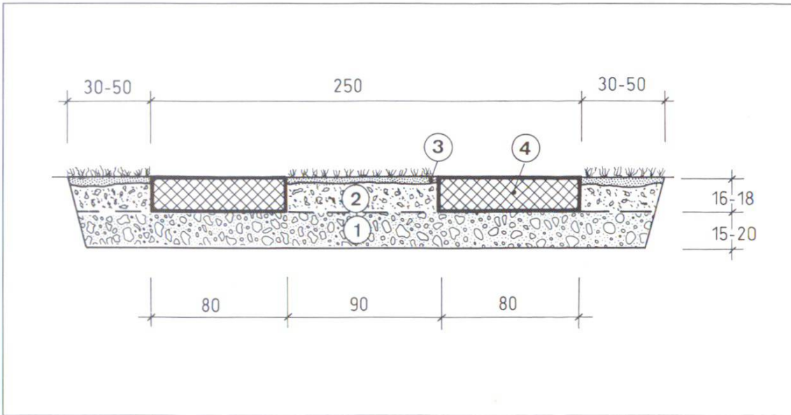
Structure schématique de bandes de roulement: (1) gravier ou pierraille pour routes (ancien ou nouveau), (2) matériau résistant à l'érosion, p. ex. grave, (3) humus, (4) béton B 35/25. (Source: BeAG, Wildegg)
