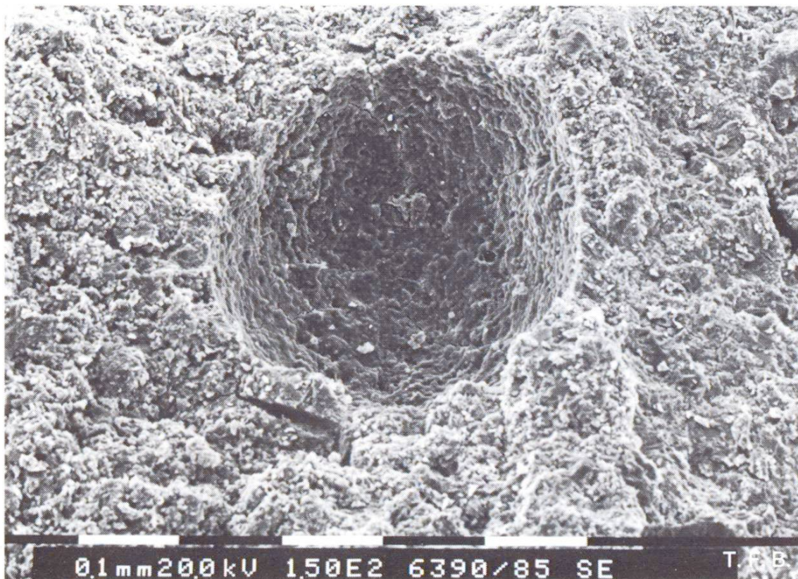
Fig. 3 Pores d'air dans une pâte de ciment de e/c = 0,50 (photo: Laboratoire de microscopie électronique de l'Université de Bâle).
