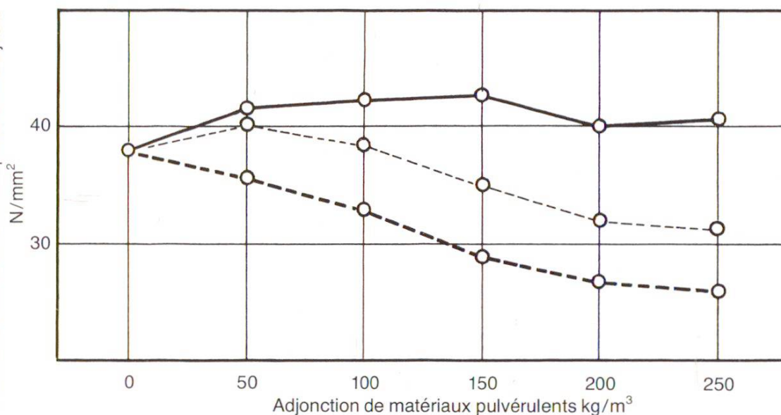
Fig. 1 Résistance à la compression d'un béton avec différents ajouts pulvérulents. Béton CP 300, 0–32 mm, plastique. Trait plein: chaux hydraulique Traitillé fin: filler «fin», 0–0,1 mm Traitillé gras: filler «gros», 0,1–0,2 mm Essais TFB 1976.
