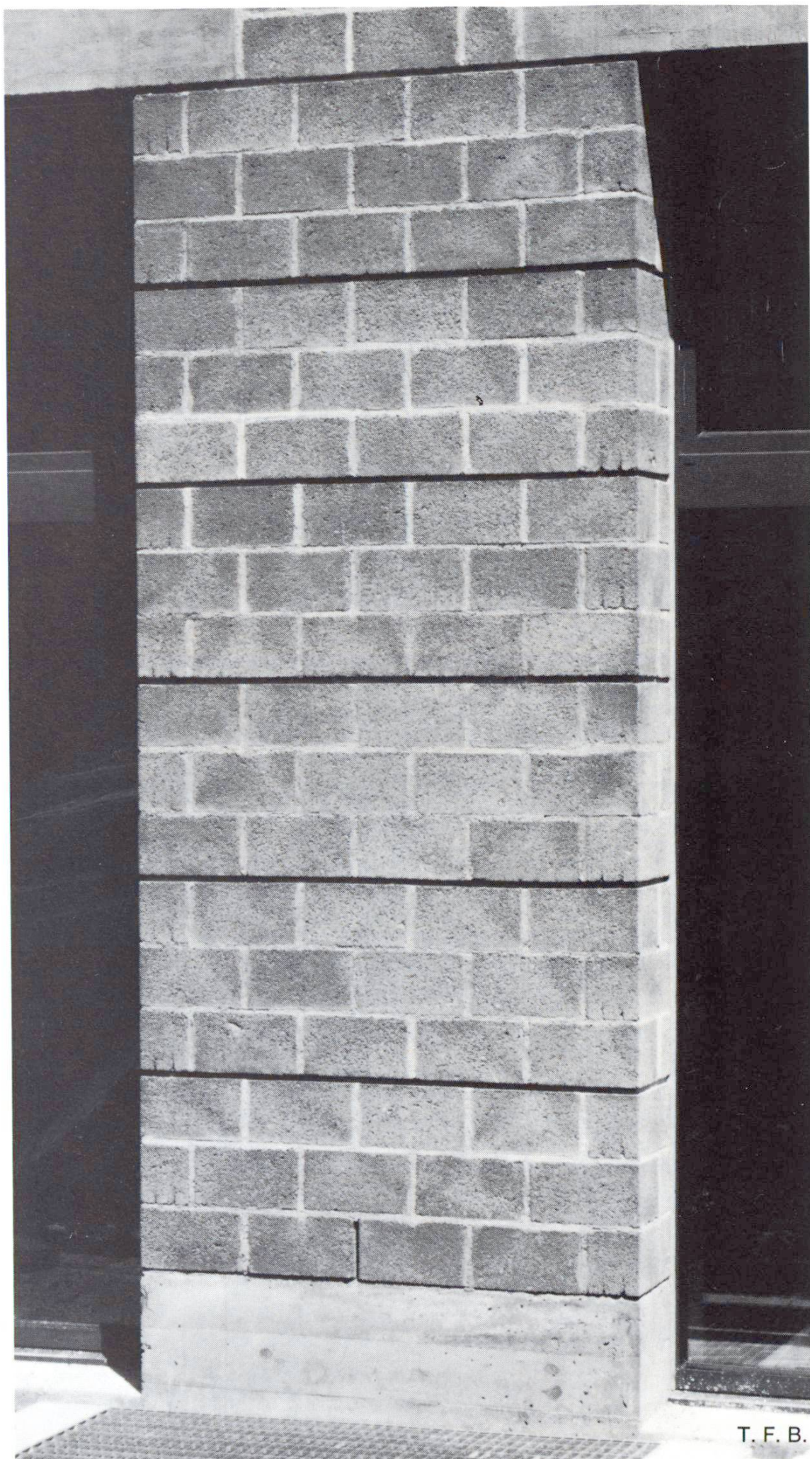
Fig. 8 Maçonnerie apparente en béton dans un assemblage spécial.
