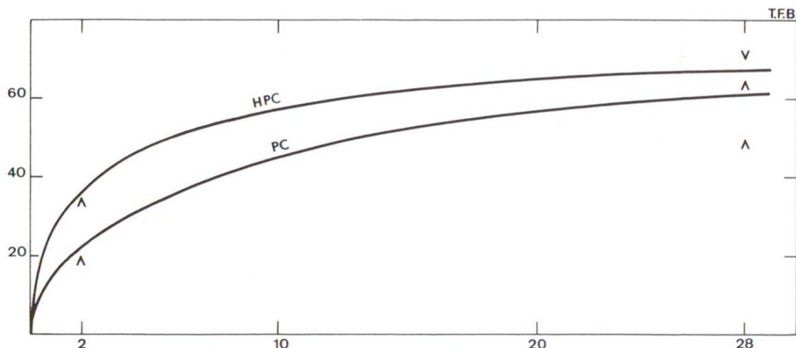
Fig. 1 Augmentation des résistances exigées par les normes pour le CP et le CPHR.
