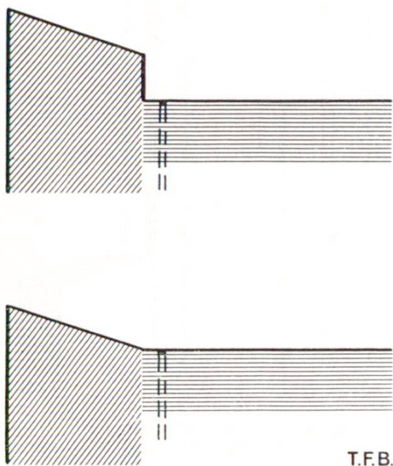
Fig. 2 Couronnement de mur au niveau de la toiture, avec pente vers l'intérieur et drainage. En bas: Mauvaise disposition, insuffisante en cas de vent venant de droite.
