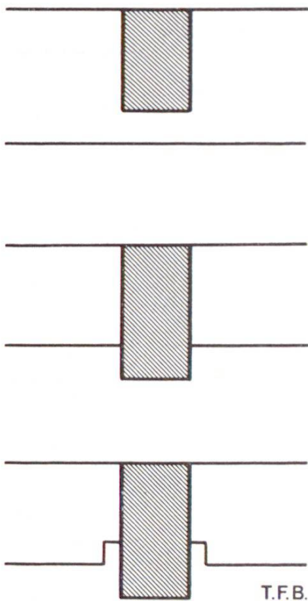
Fig. 3 Croisement entre montant et tablette (vue en plan). En haut: mauvais. Au milieu: mieux. En bas: bon.
