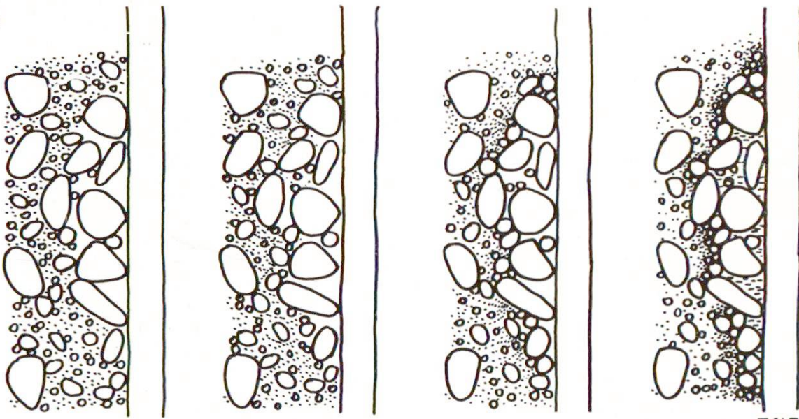
Fig. 2 Dans le mouvement du mortier vers un nid de gravier, il peut se former une structure filtrante dans laquelle des grains obturent le passage des suivants. En pareil cas, seule l'eau peut encore pénétrer dans les vides où elle délave les grains de gravier et remonte le long du coffrage (fig. 7 et 8)
