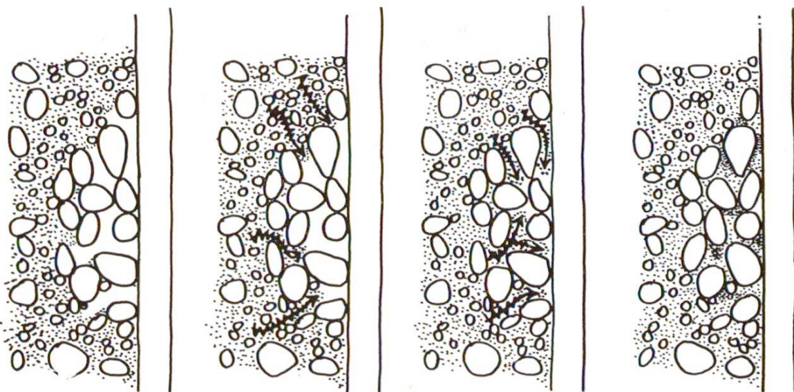
Fig. 1 La vibration du béton frais provoque un écoulement du mortier vers les vides des nids de gravier. L'arrêt de la vibration stoppe le processus. A la surface des bétons, on peut donc observer tous les stades de cette « guérison ». Dans le mortier en mouvement la répartition de l'eau et du ciment est souvent inégale, ce qui se manifeste par des teintes claires et foncées en forme de nuages (fig. 4).
