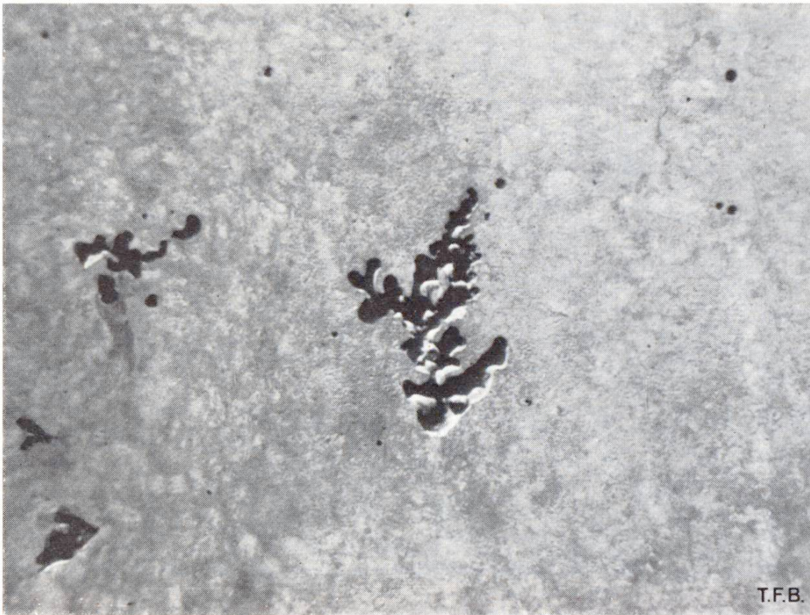
Fig. 6 Nid de gravier partiellement colmaté, le long d'un coffrage lisse et bien étanche. Si la vibration avait duré plus longtemps, on aurait probablement eu une accumulation de bulles d'air.
