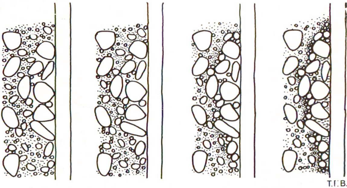
Fig. 2 Dans le mouvement du mortier vers un nid de gravier, il peut se former une structure filtrante dans laquelle des grains obturent le passage des suivants. En pareil cas, seule l'eau peut encore pénétrer dans les vides où elle délave les grains de gravier et remonte le long du coffrage (fig. 7 et 8)
