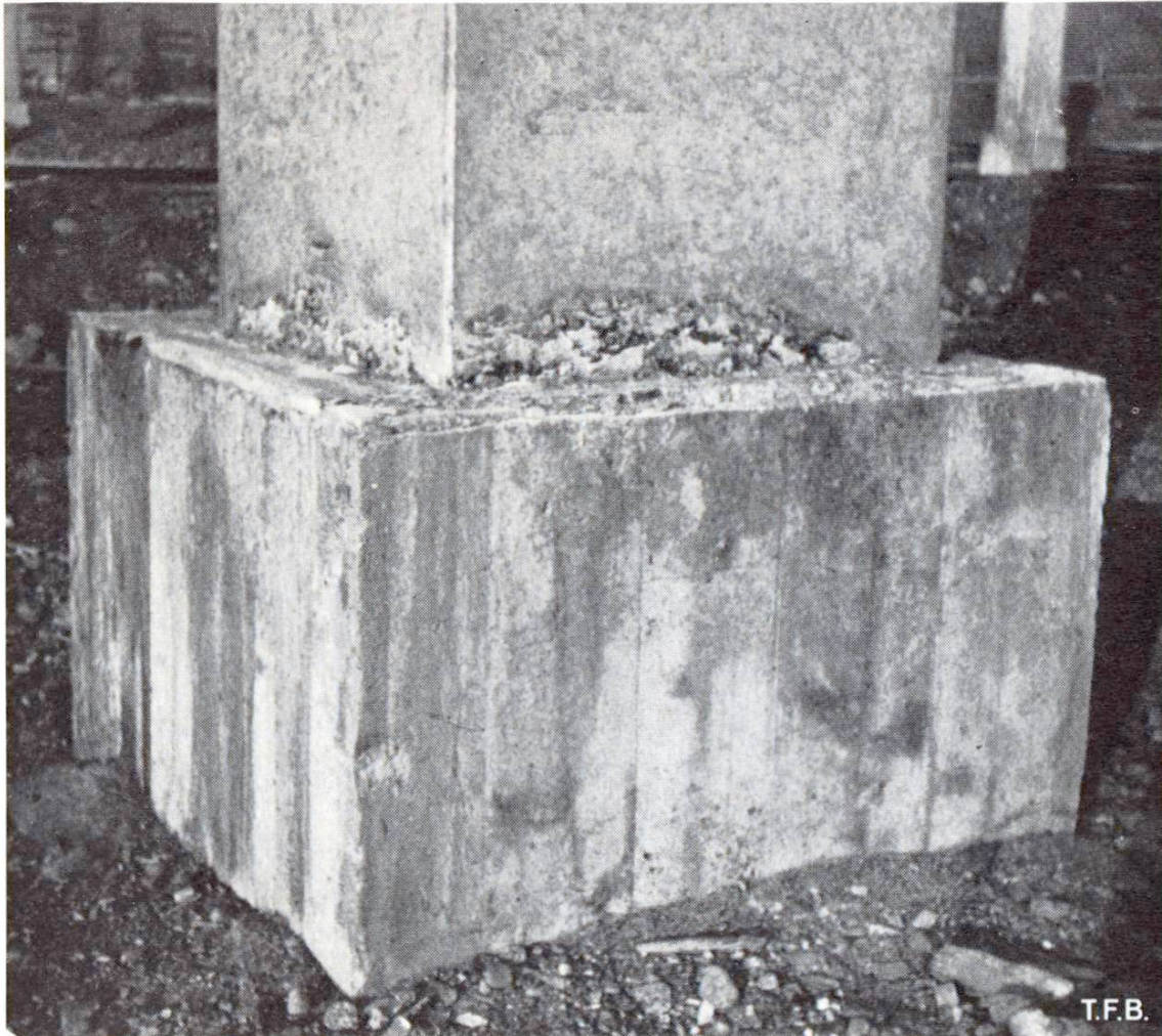
Fig. 7 Nid de gravier au pied d'un pilier (grande hauteur de chute) avec formation d'une structure filtrante et délavage des grains de gravier par l'eau. Cet effet a encore été aggravé par des joints de coffrage non étanches.
