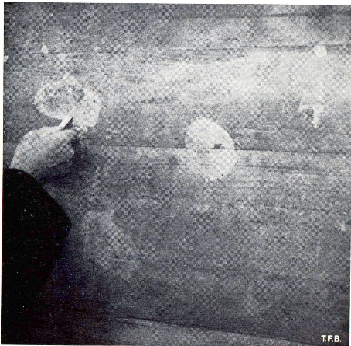
Fig. 5 Une absorption irrégulière de l'eau du béton par le coffrage provoque des variations locales du facteur eau:ciment. Des nœuds de ce panneau de coffrage ont été enlevés et remplacés par du bois normal; les zones où la colle a coulé ont absorbé moins d'eau que les autres.
