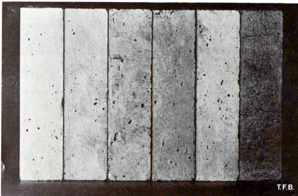
Fig. 1 Divers tons de gris d'un béton provoquées par des différences dans les conditions de conservation. (Les éprouvettes ont toutes été préparées de la même façon et ont exactement la même composition).
