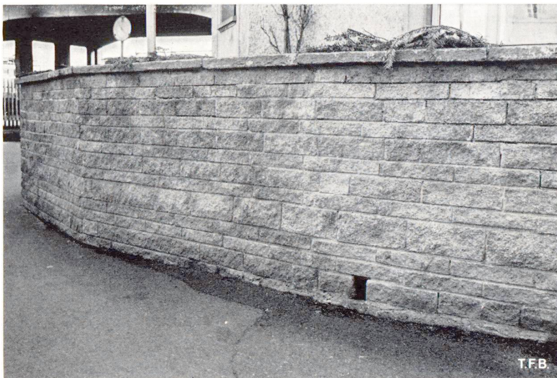
Fig. 2 Revêtement à assises parallèles irrégulières.
