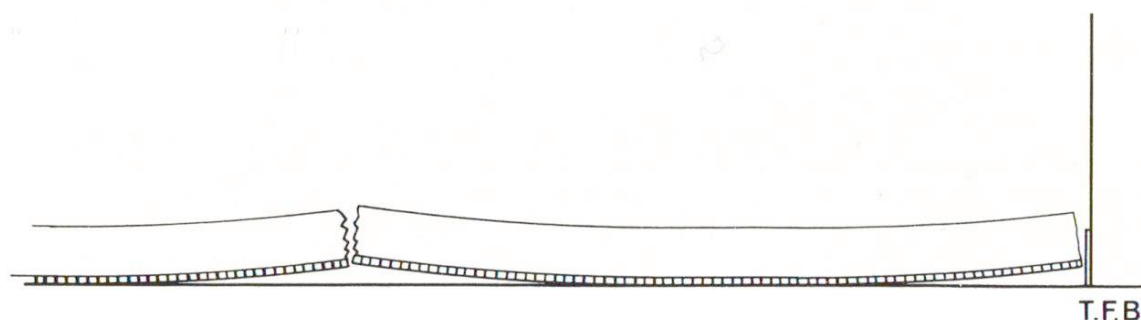
Fig. 5 Un desséchement trop rapide du béton de chape entraîne la formation de fissures de retrait. Il provoque aussi un plus grand raccourcissement de la surface supérieure et une tendance au gauchissement de la chape le long des fissures et des bords.
