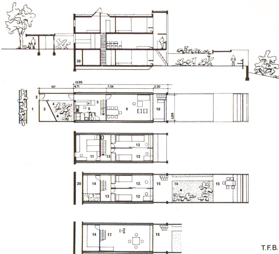
Fig. 3 Plans d'une maison du type 380
