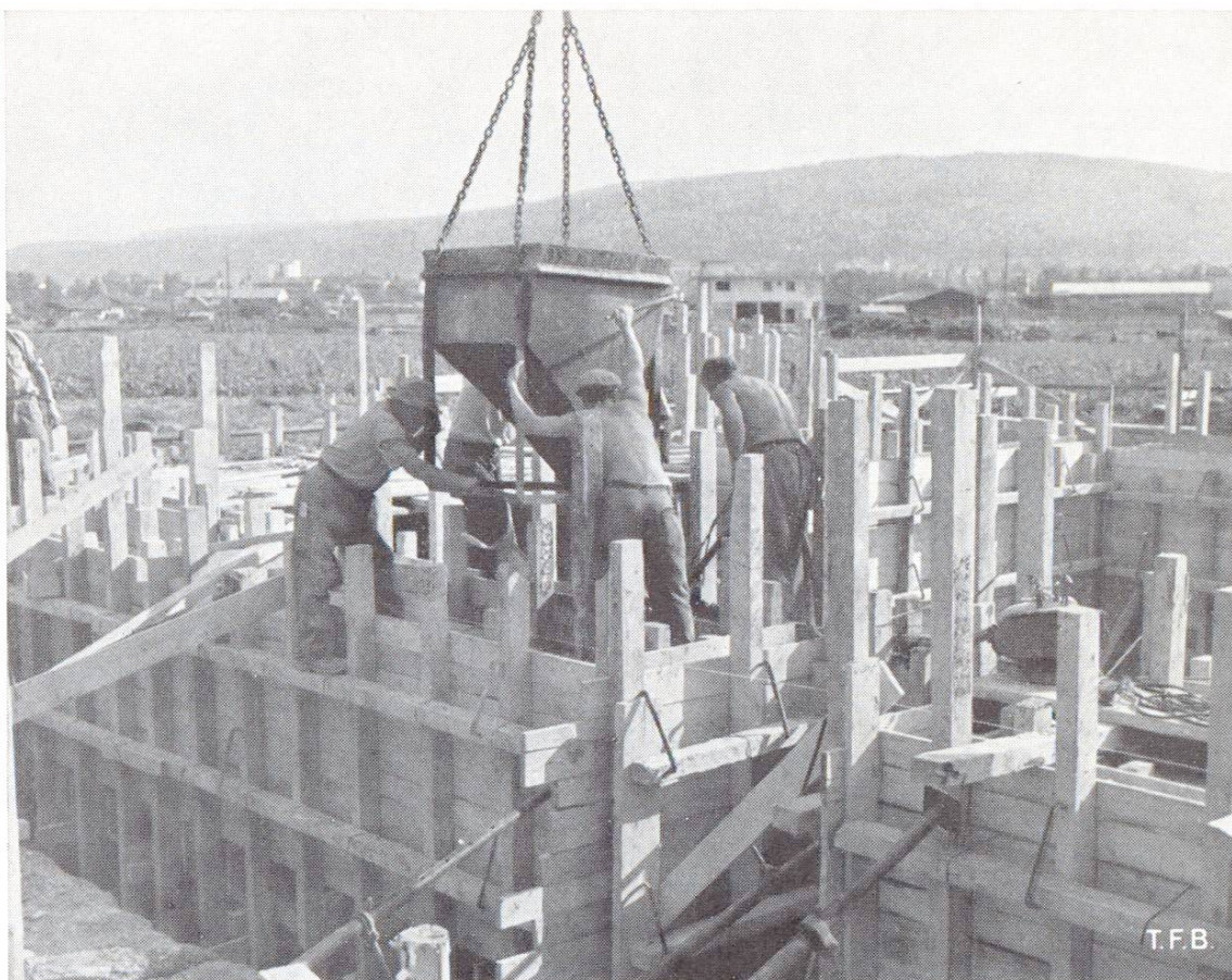
Fig. 5 Le déversement direct des bennes de transport n'est admissible que pour de faibles hauteurs de chute et dans les constructions de dalles ou de gros ouvrages. La photo montre une telle opération faite dans un cas qui ne remplit pas ces conditions
