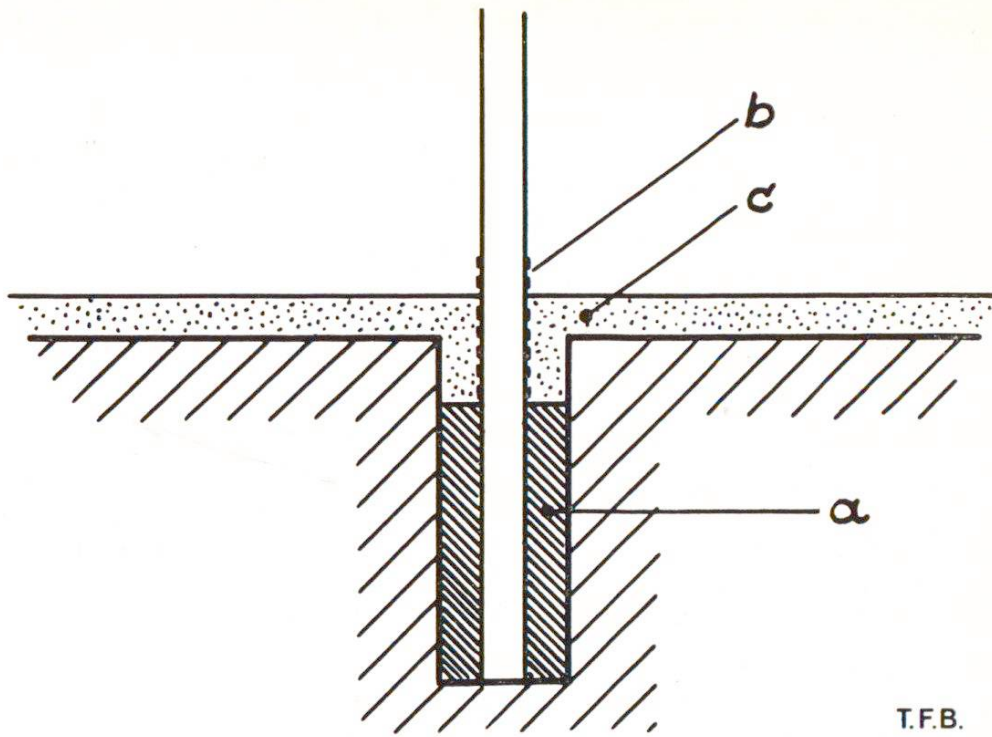
Scellement d'un montant en fer dans un mur de béton. a) mortier à prise rapide, b) badigeon au lait de ciment, c) enduit
