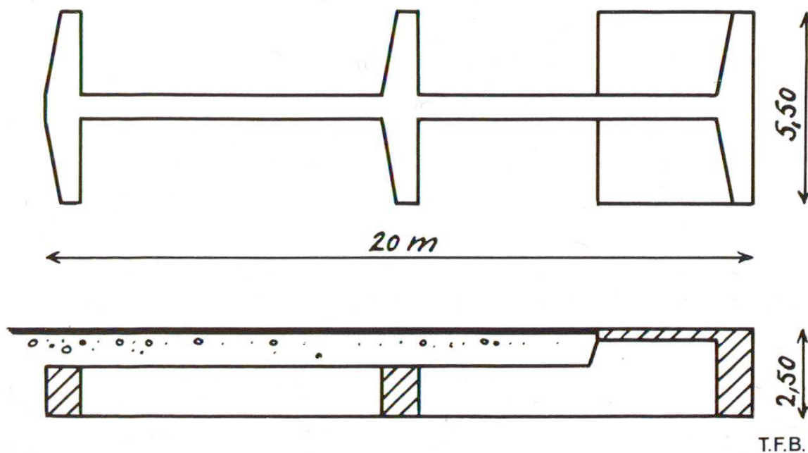
Fig. 6 Plan et coupe de la culée
