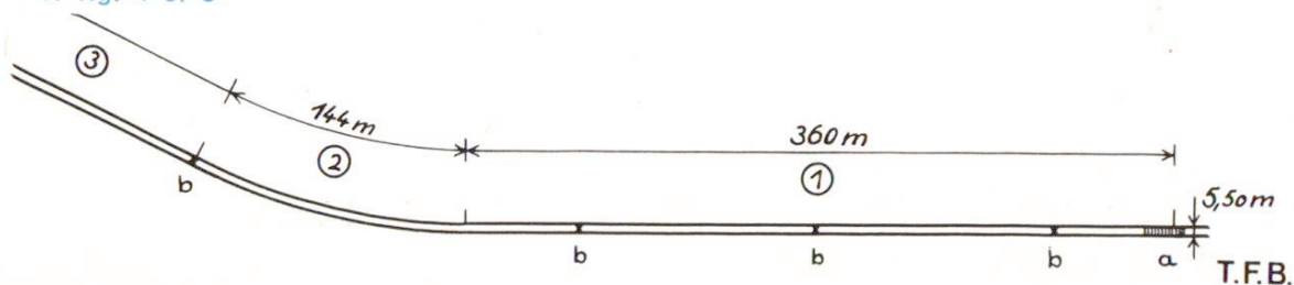
Fig. 3 Route expérimentale en béton précontraint entre Möriken et Brunegg 1) Tronçon rectiligne, dalle de 12 cm d'épaisseur 2) Tronçon précontraint en courbe, dalle de 15 cm d'épaisseur (Coupe fig. 7) 3) Tronçon dans lequel la poussée de la précontrainte est absorbée progressivement par une route en béton classique, a) culée, v. fig. 6, b) Coins, v. fig. 4 et 5
