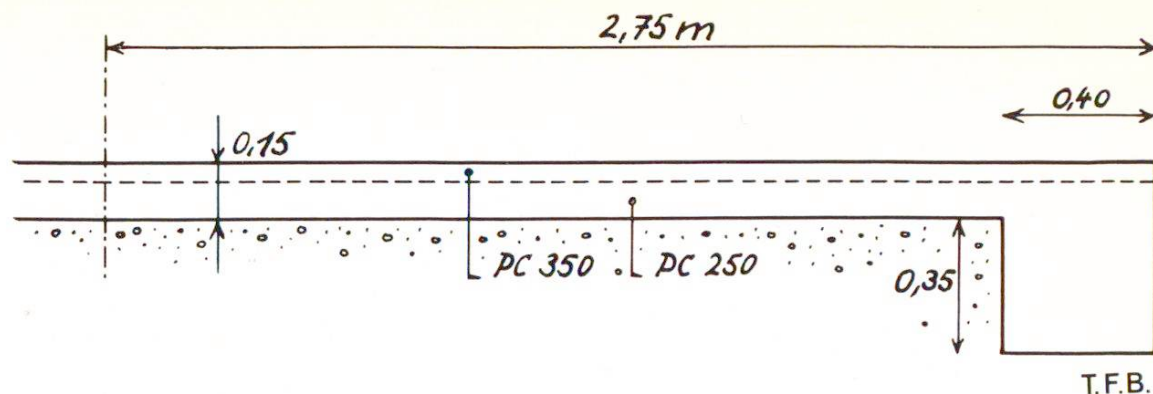
Fig. 7 Coupe transversale du tronçon précontraint en courbe avec son éperon de 35 cm du côté intérieur de la courbe
