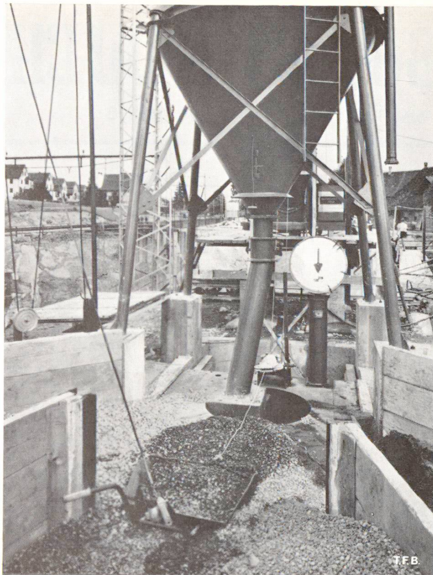
Fig. 1 Installation moderne de préparation du béton avec agrégat livré en trois composants et dosage pondéral
