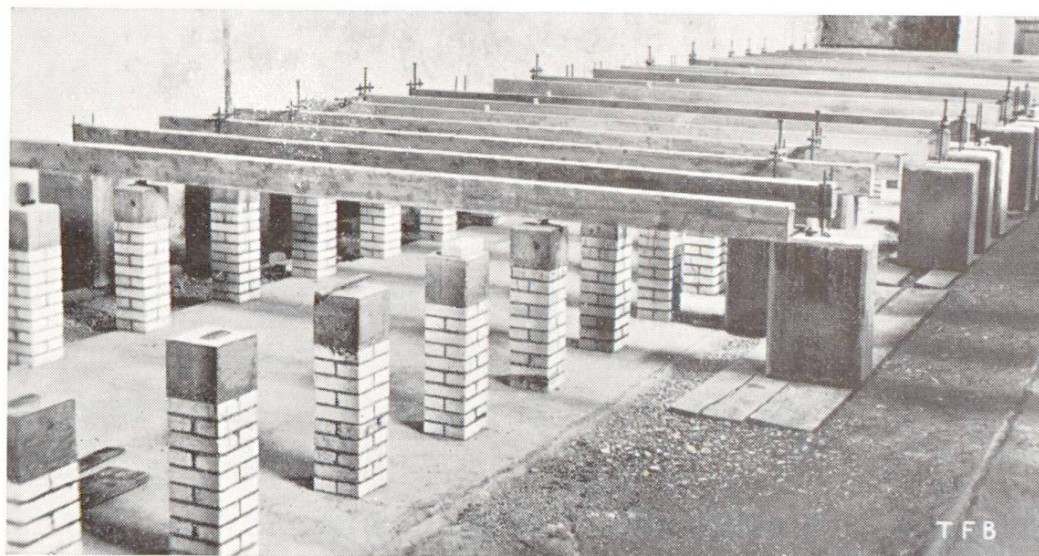
Fig. 3 Poutres d'essai en béton précontraint. Essais organisés par la S. I. A. en 1941
