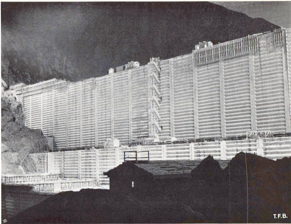
Fig. 6 Barrage de la Grande Dixence. Etat des travaux en août 1957. Environ 2,5 millions de mètres cube de béton
