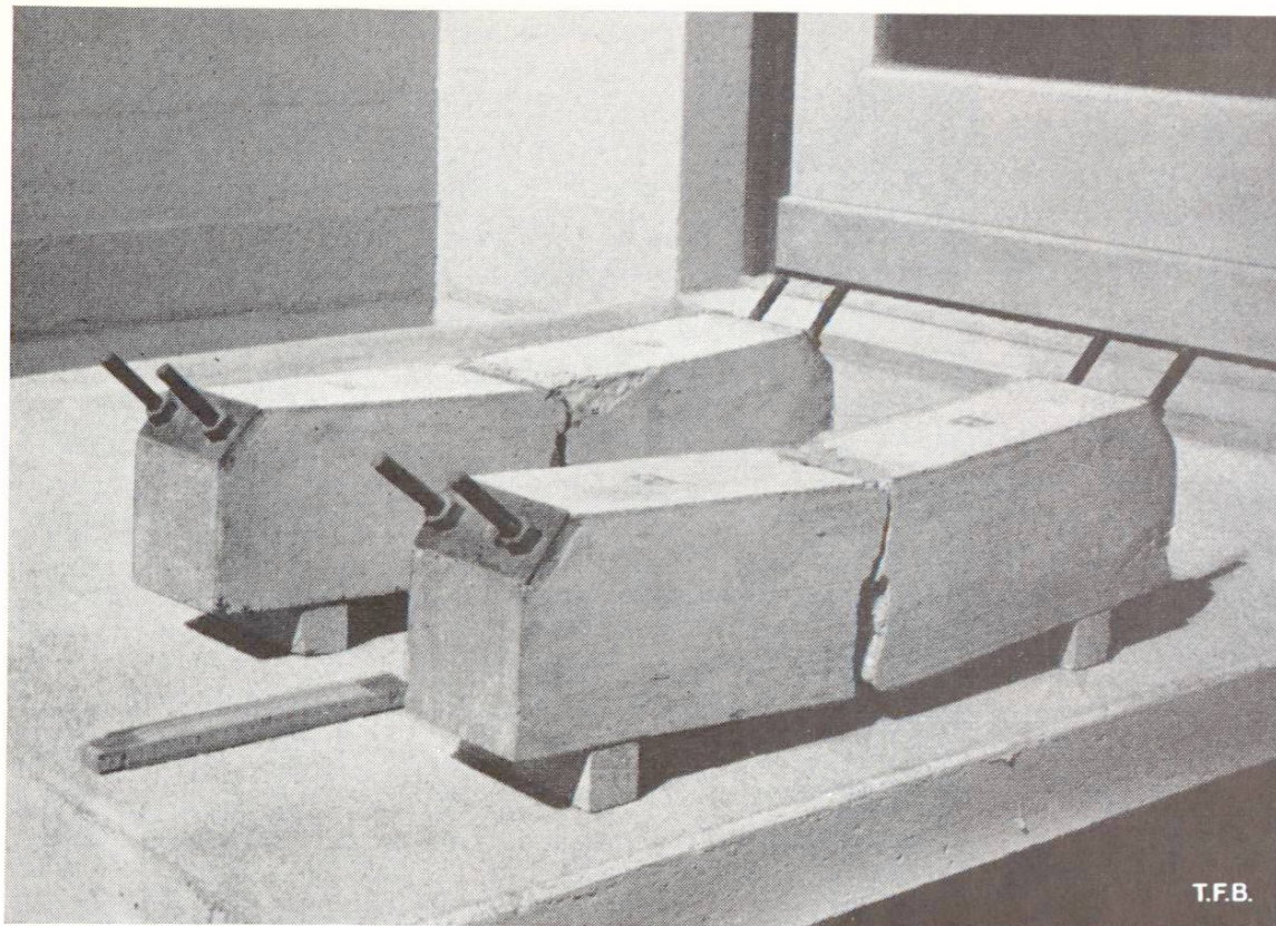
Fig. 2 Prismes d'essai en béton précontraint fabriqués en 1940 par le T. F. B.
