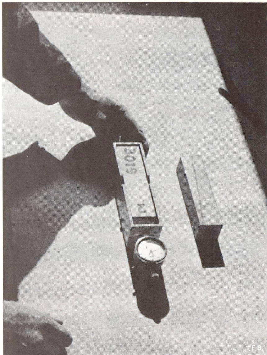
Fig. 4 Mesures de retrait sur des prismes de mortier normal selon une méthode simplifiée mise au point par le T. F. B.
