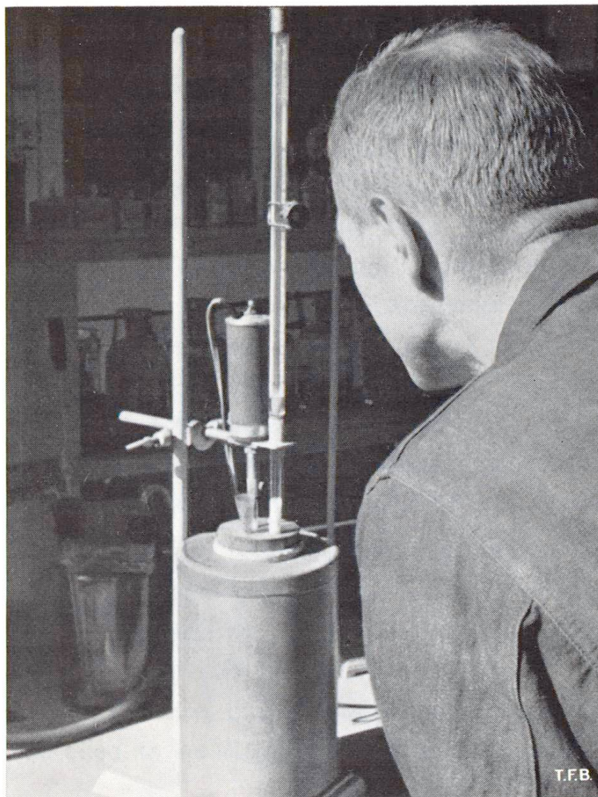
Fig. 5 Détermination de la chaleur de solution du ciment portland au laboratoire du T. F. B.
