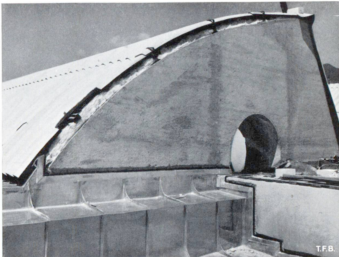
Fig. 10 Détail de l'isolation thermique extérieure recouverte en éternit ondulé, construction simple et économique
