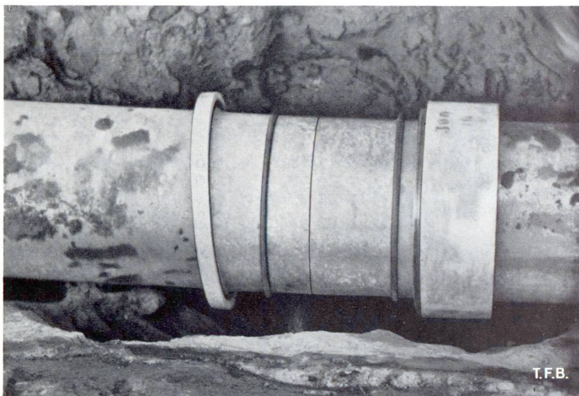
Fig. 6 Positions du manchon, du collier et des anneaux avant le montage
