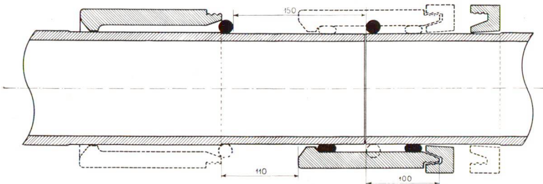
Fig. 4 Le nouveau joint „Simplex” avec collier à vis. Le principe de l'étanchéité est le même qu'à la figure 2
