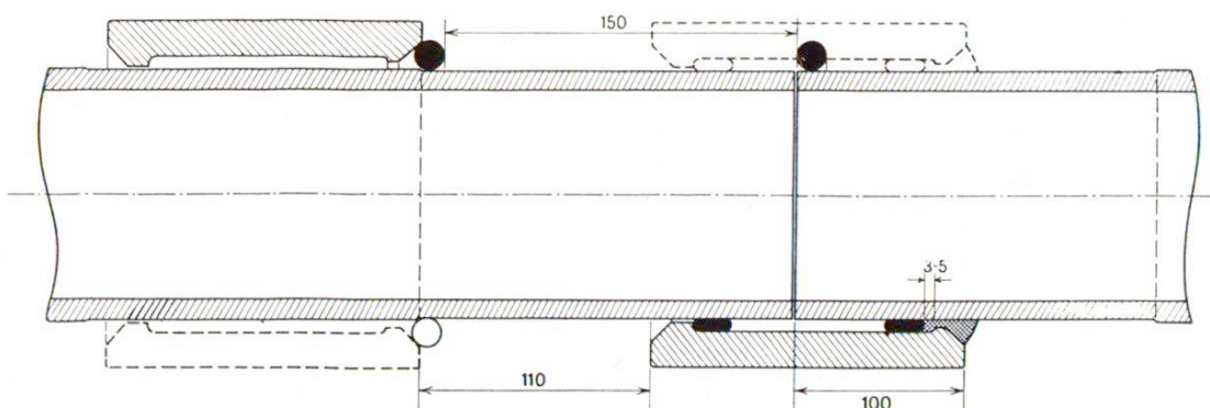
Fig. 2 Coupe du joint „Simplex”. On y voit la position du manchon et des anneaux de caoutchouc avant et après le montage. Hachuré croisé, le bouchon de mortier indispensable
