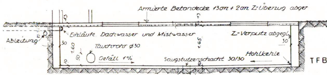
Fig. 1 et 2 Fosse à purin de 40 m³. Plan et coupe longitudinale
