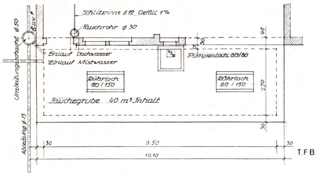
Längsschnitt
