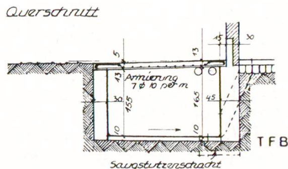
Fig. 4 Coupe transversale de la fosse à purin Querschnitt = Coupe transversale Armierung = armature 7 \phi 10 per m = 7 \phi 10 par m. c. Saugstutzenschacht = puisard
