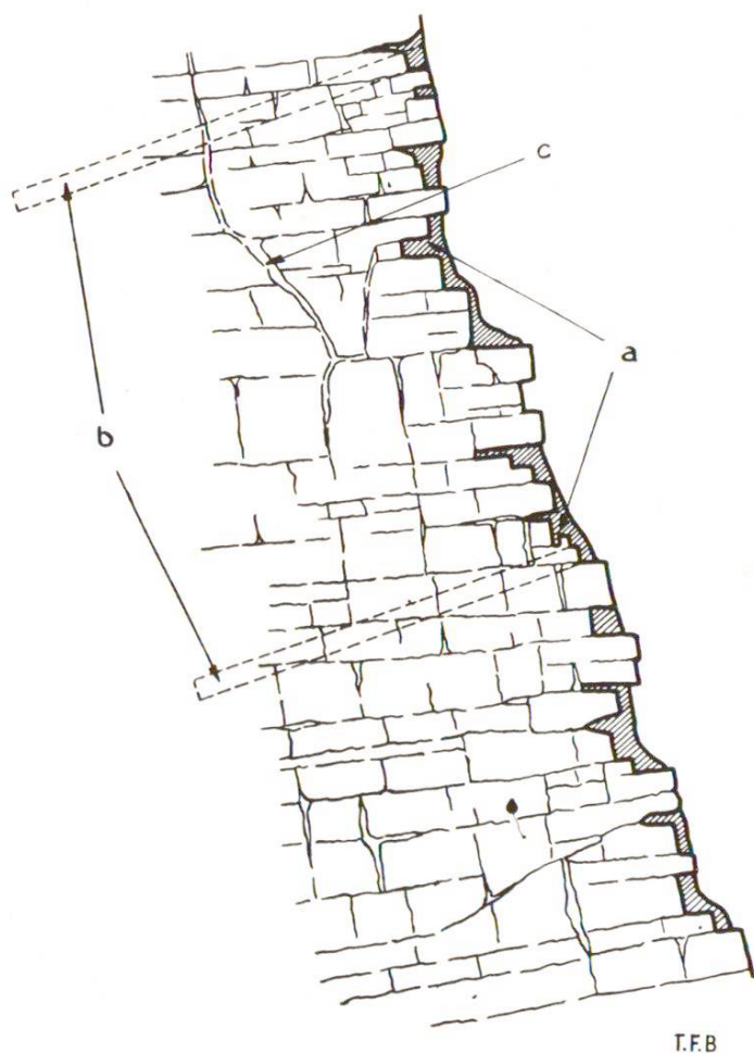
Fig. 3 Consolidation d'une raide paroi de rocher
