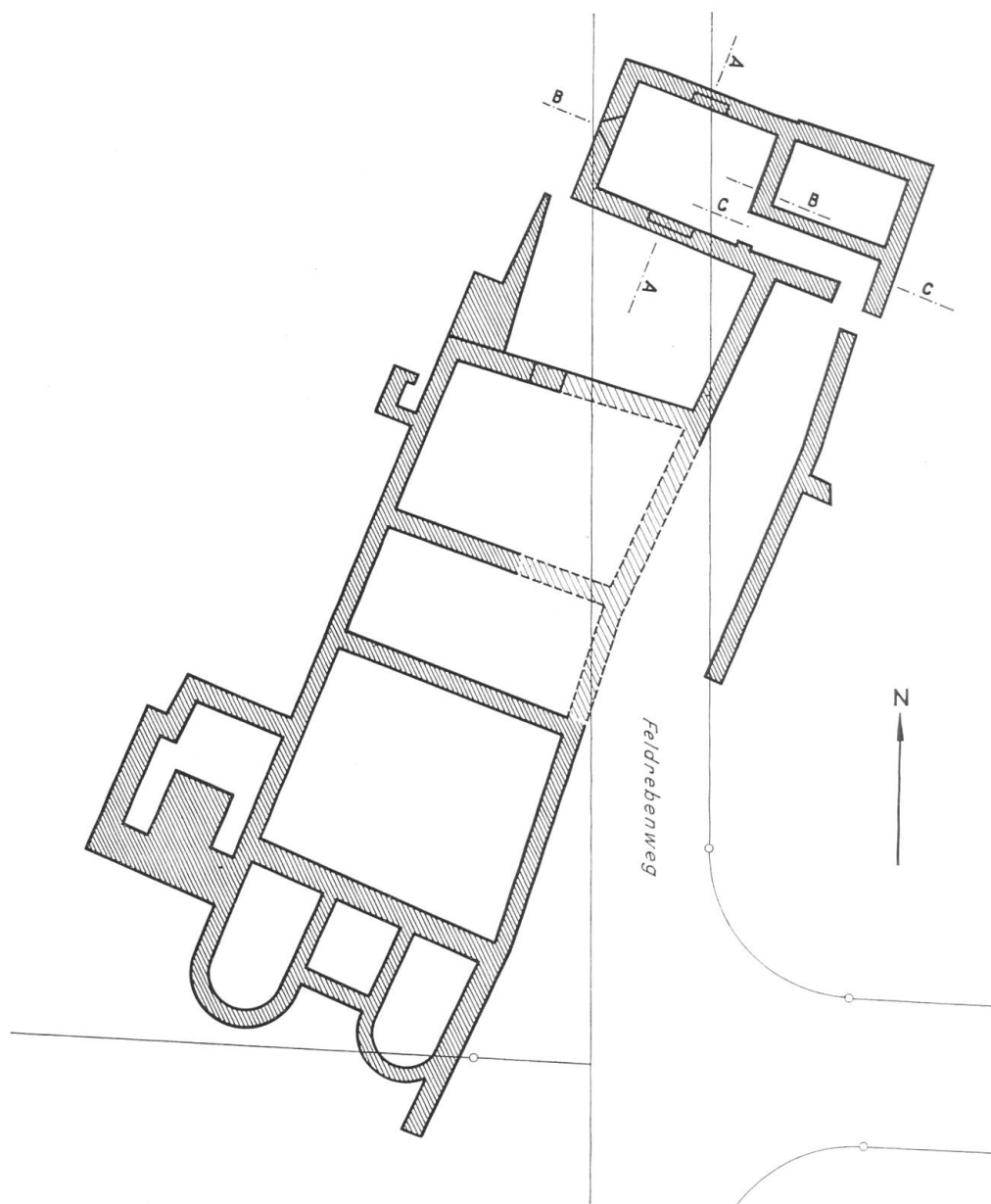
Bild 2. Grundriss der Villa in den Feldreben, Muttens. Aus Baselbieter Heimatbuch 8, S. 161. — Auf der NNE-Schmalseite der 1957 freigelegte Keller mit Treppenanlage.
