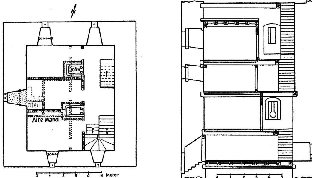
Abb. 12 Im Archiv des Bauamtes Baden liegen Pläne im Maßstab 1:50, die Architekt Adolf Blum 1869 resp. 1873 für den Einbau von Gefängniszellen in den Wylerturm (= Bruggerturm) gezeichnet hat. – Einer (von 1869) zeigt für den 3. und 4. Boden je drei Zellen, die durch Doppelholzwände von einander getrennt und durch Kantholzwände gegen den Gang abgeschlossen sind. Je zwei Zellen sind heizbar, die dritte nicht. – Die vier Pläne von 1873 zeigen ähnliche Abgrenzung wie im Plan von 1869, außerdem eine Variante mit Trennung der Zellen durch gemauerte Wände. In einer Variante ist Einzelheizung der Zellen, in der anderen Zentralheizung vom ersten Boden aus vorgesehen. Diese wurde später ausgeführt und nach 1900 alle Wände mit Eternitplatten verschalt.
