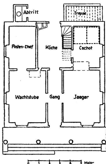
Abb. 13 Landjägerposten an der Bruggerstraße. Ausschnitt und Umzeichnung des Stiches von Mayer-Attenhofer, 1853, und Grundriß von Adolf Blum 1870.
