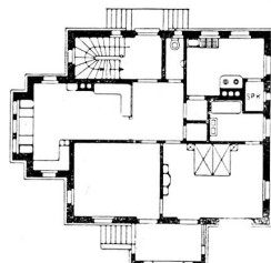
Villa Naef à Küsnacht (Zurich). — Plans 1 : 400. — Architecte: O. Honegger, Zurich.
