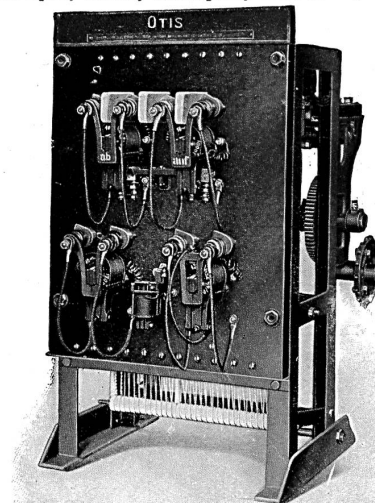
Contrôleur magnétique
