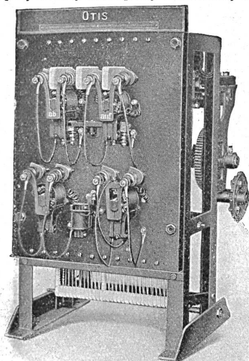
Contrôleur magnétique
