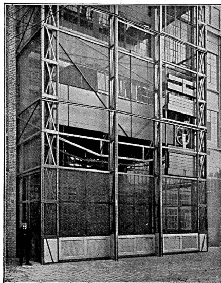
Ascenseur automobile
