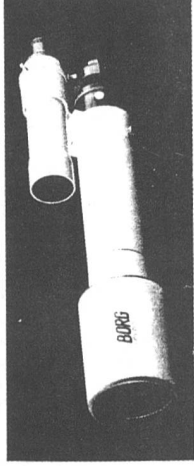
Borg 100 f640 HA; 2,2 kg Borg 100 f640 ED; 2,2 kg
