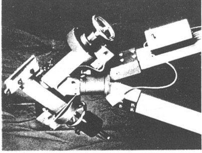
Goliath incl. 2-Achsensteuerung und Dreibeinstativ
