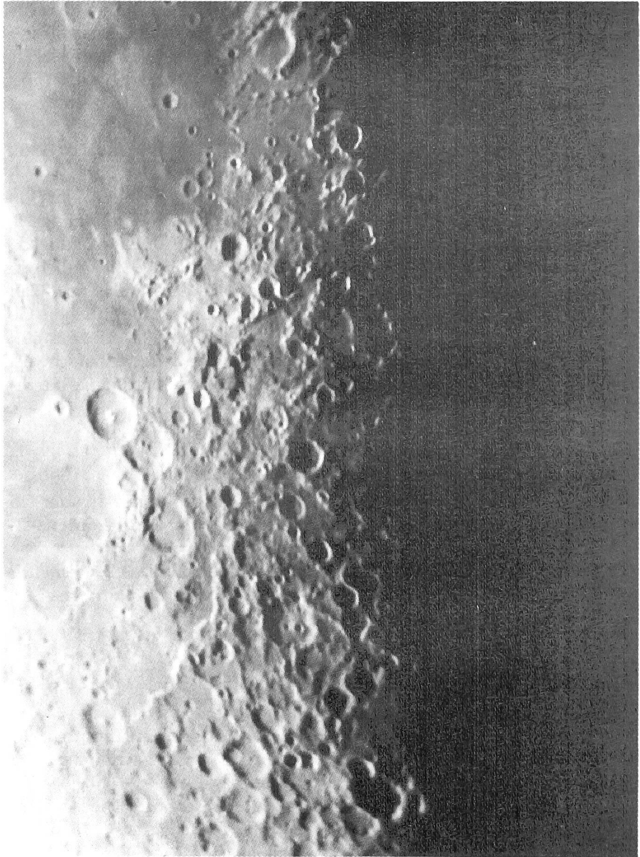
Region um den Mondkrater Theophilus. Meade 25 cm Schmidt-Cassegrain Teleskop, Äquivalentbrennweite 9 m. \frac{1}{4} s belichtet auf Ilford Delta 400, entwickelt in Microphen. Aufnahme von Rouven Lüscher, Rapperswil.
