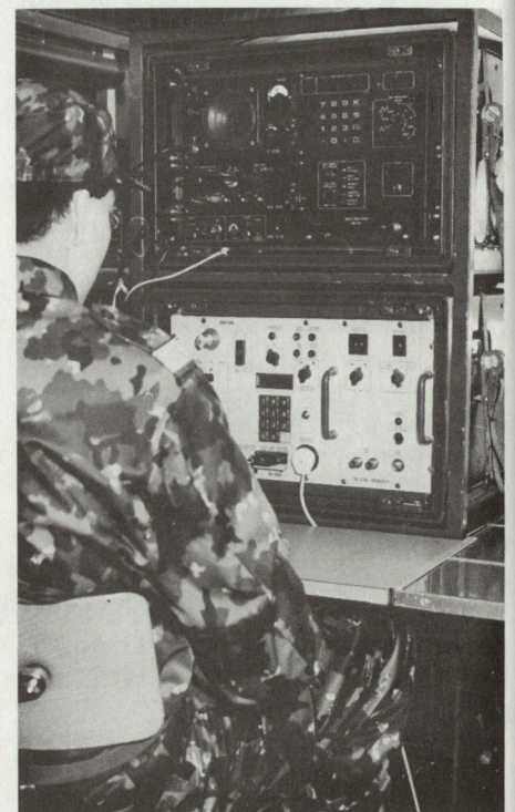
Die Kommandofunkstation SE-430 mit Chiffriergerät TC-535.
