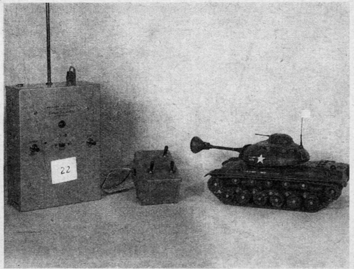
Bild 1. Das Bild zeigt rechts ein ferngesteuertes Modell des M48A2-Panzers im Maßstab 1:25. Ganz links ist der Sender ersichtlich, der zugleich die Bedienungsschalter für die Raupenkettens enthält. In der Mitte ist das Kontrollgerät für Turm und Kanone zu sehen
