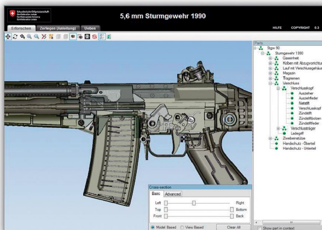
3D-Lektion Sturmgewehr 90, erstellt mit der Software NGrain.
