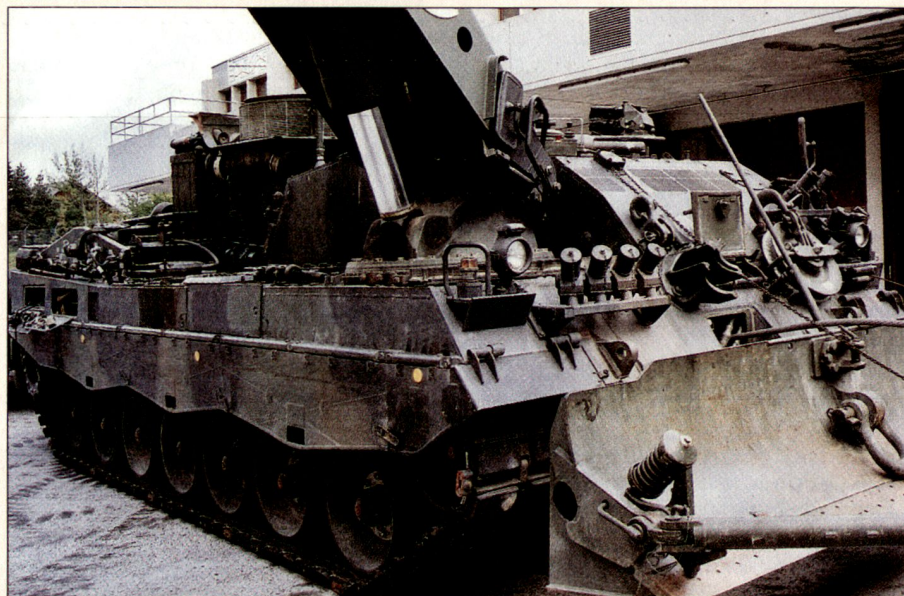
Bergepanzer.
