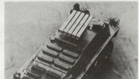
Bild 2: Wannenoberdeck des BRDM-2 mit AT-5/Spandrel-Abschussrohren
