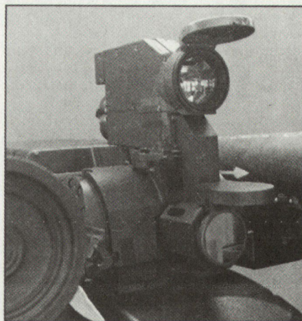
Zur Kampfwertsteigerung erhält MILAN (wie auch Projekt HOT) einen Gefechtskopf mit höherer Durchschlagsleistung und voller Kompatibilität zur bisherigen Anlage.
