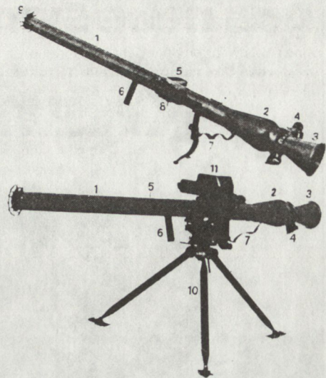
1 Lauf, 2 Zündungskammer, 3 Düse, 4 Verbindungsklammer, 5 Abzug, 6 Abzugsicherung, 7 Schulterstütze, 8 Zielvorrichtung, 9 Mündungsbremse, 10 Dreifuss, 11 Zielvorrichtung mit Entfernungsmesser
