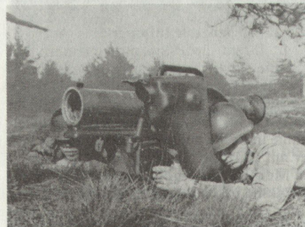
Bild 17: Hauptproblem Panzerabwehr
