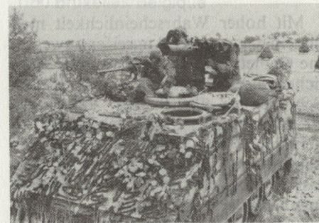
Bild 19: Hauptproblem Panzerabwehr
