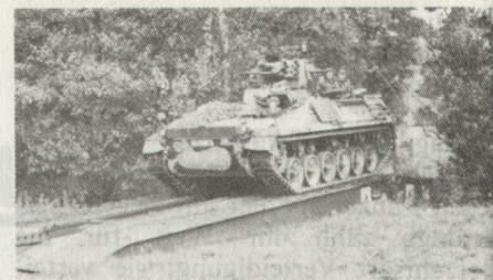
Bild 9: Gepanzerte Infanterie
