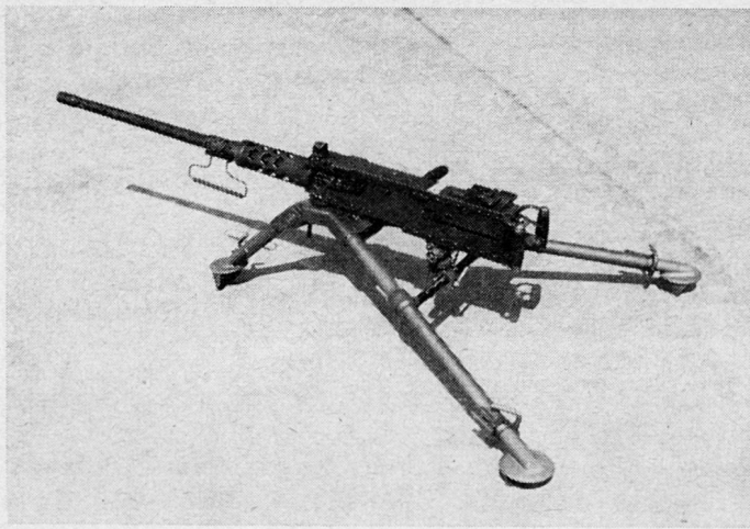
Bild 2. 12,7-mm-Maschinengewehr 64, auf der Dreibeinlafette montiert. Diese Einsatzart dürfte die Ausnahme sein, wiegen doch Waffe und Lafette zusammen rund 48 kg. Der Aufwand dieses Einsatzes lohnt sich höchstens in stabilen Verhältnissen.
