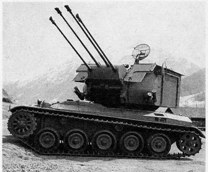
Bild 2. Prototyp eines schweizerischen Flabpanzers auf Chassis AMX mit Oerlikon-20-mm-Vierling
