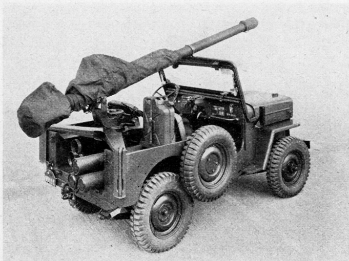
106-mm-BAT, Aufbau auf Jeep
