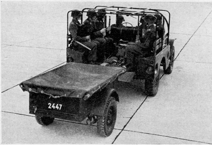
Bild 2. Motordragoner-Minenwerfergruppe aufgesessen
