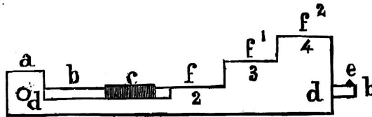
a Pivot. d d Visierfuss mit Backe. b b Leiter. e Kimme des Standvisiers. c Schieber. f f¹ f² Treppenstufen.
