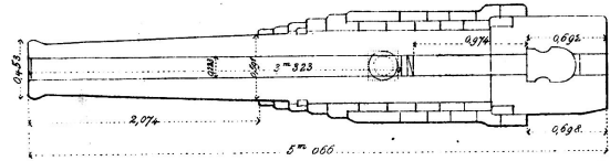
Gezogene Küstenkanone vom Kaliber von 0 m 223 (8 \frac{1}{4} englische Zolle)
